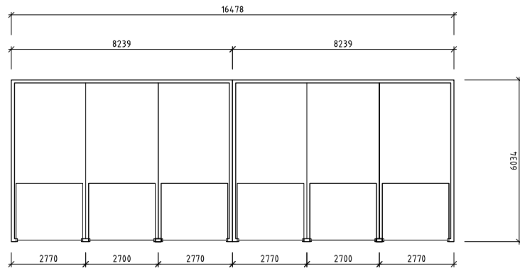
PLAN 1:100
