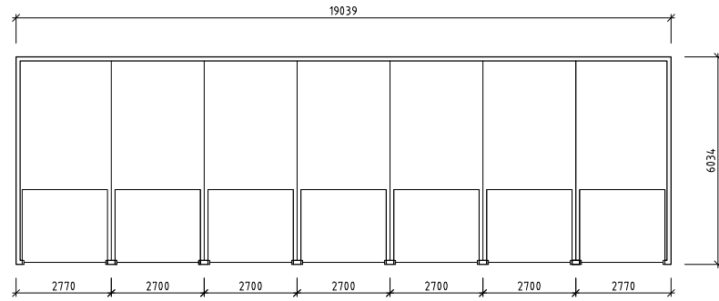
PLAN 1:100
